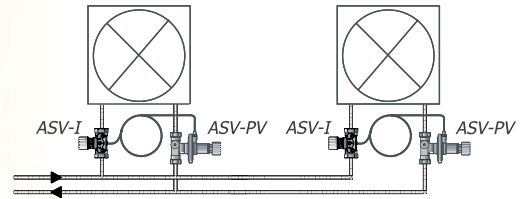
Рис. 1. Схема об'язки нагрівальних або охолоджувальних вентиляторних конвекторів (fan coils)
